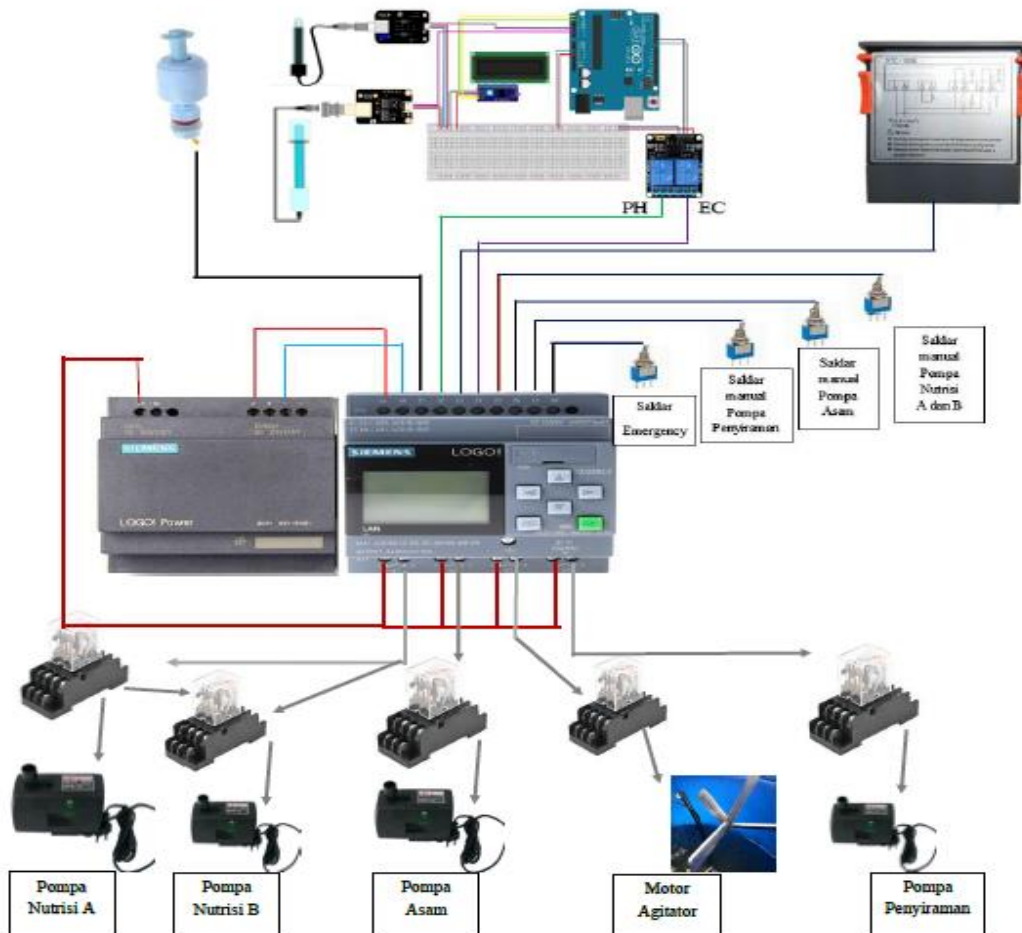
Gambar 2 Rangkaian PLC Siemens keseluruhan
